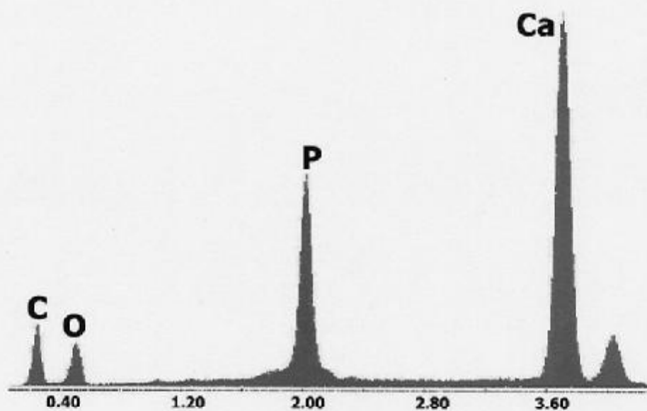
Fig. 4 – Spettro EDS relativo a osso lamellare in prossimità dell'impianto dentario.
