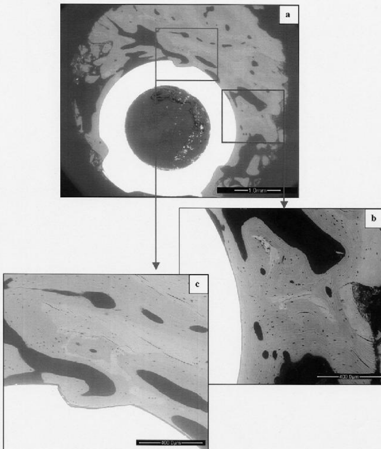
Fig. 2a, b, c – Immagine al SEM di una sezione di impianto dentario. Si nota la presenza di osso che circonda tutto l'impianto ed arriva a stretto contatto con il materiale stesso.
